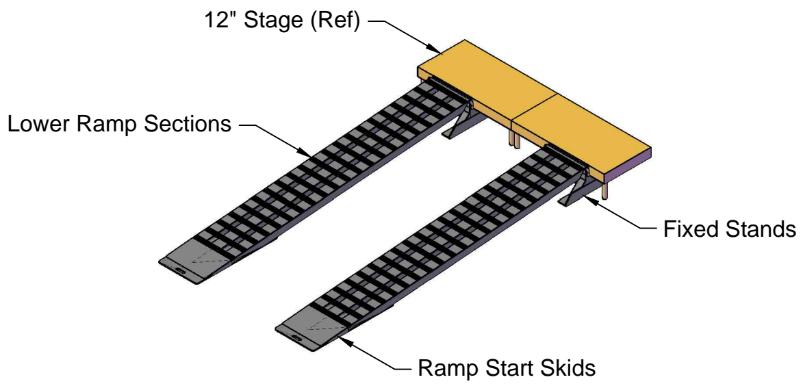
3 ISO VIEW Scale: 1/4" = 1'-0"
